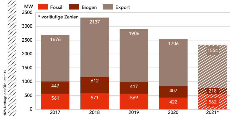
Grafik 1: Absatz von Motoren-BHKW
