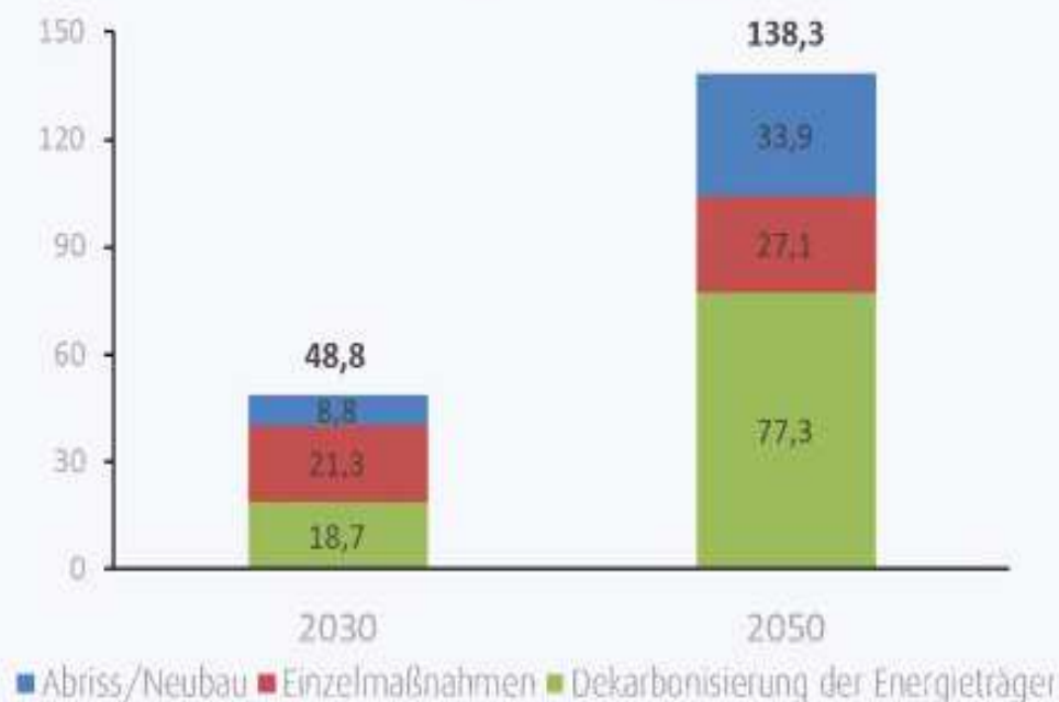
CO 2 -Einsparung in Mio. t ggü. 2020
